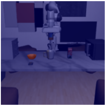
DINO+CLIP
